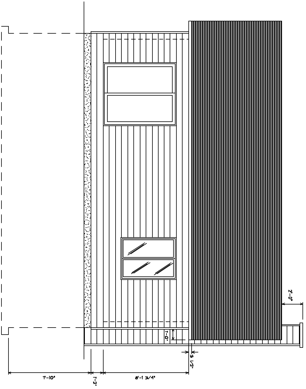
Elevation arriere
