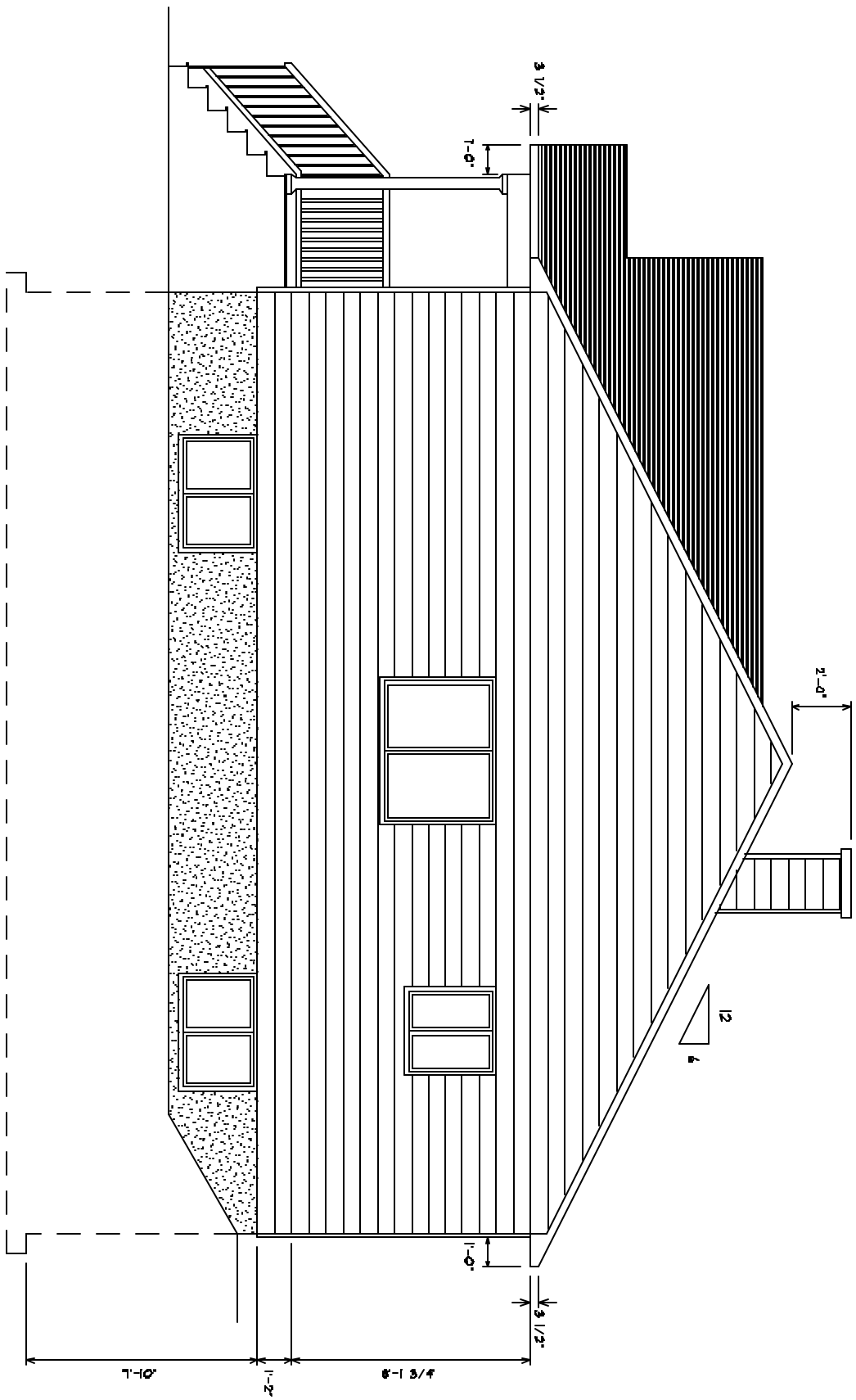
Elevation droite
