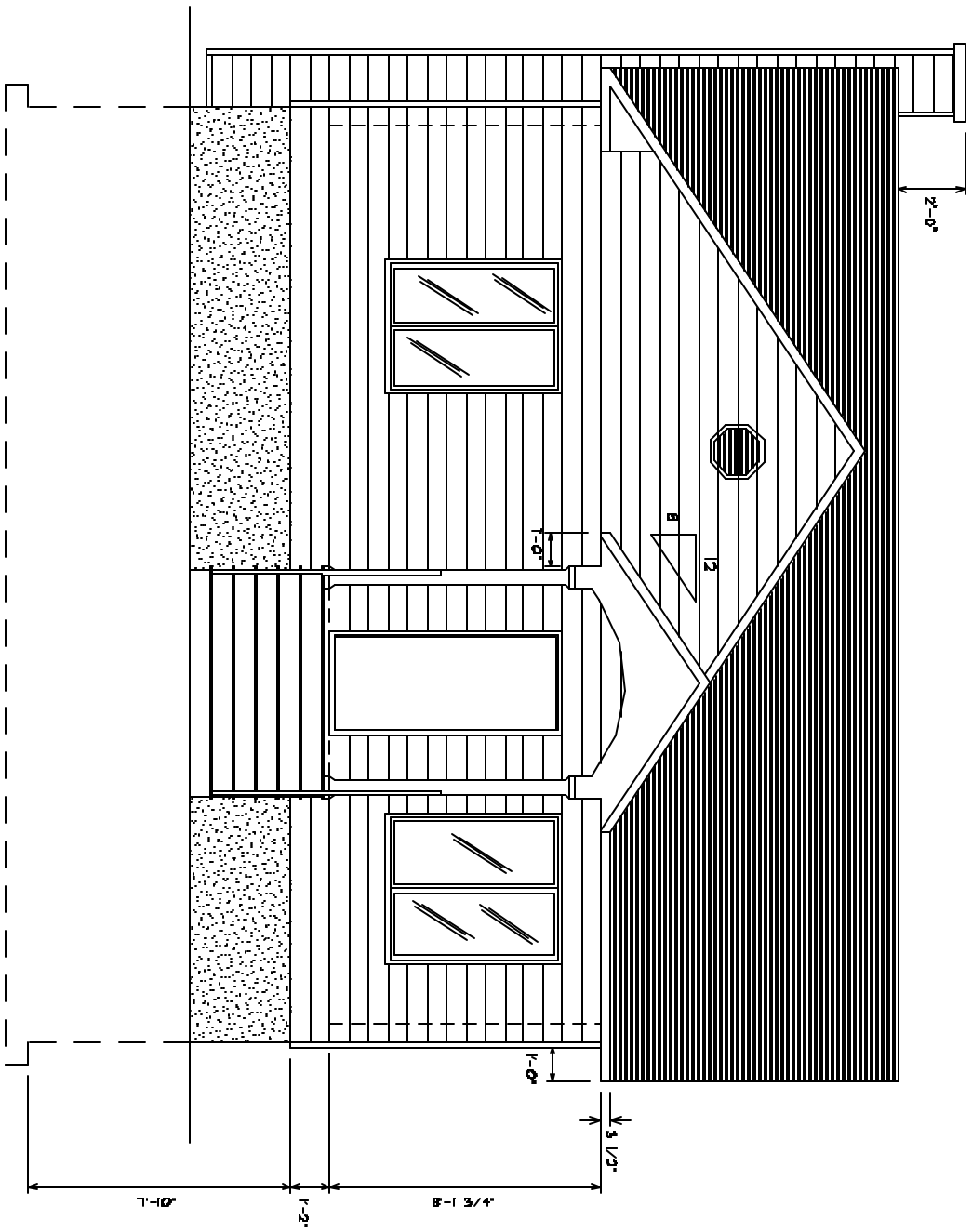
Elevation avant
