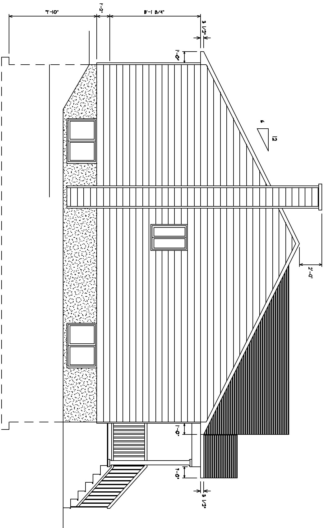
Elevation gauche
