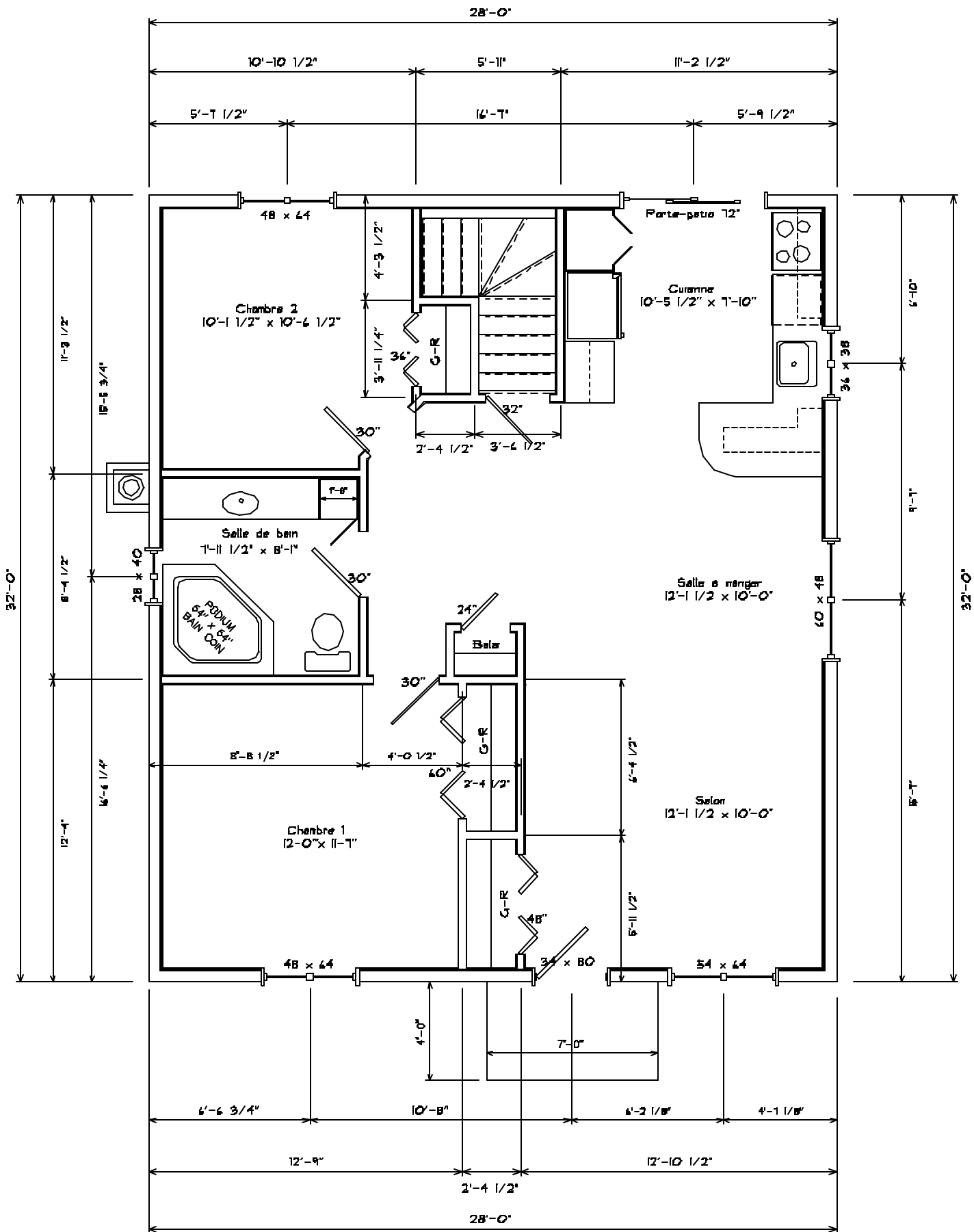
Plan de rez-de-chausée
